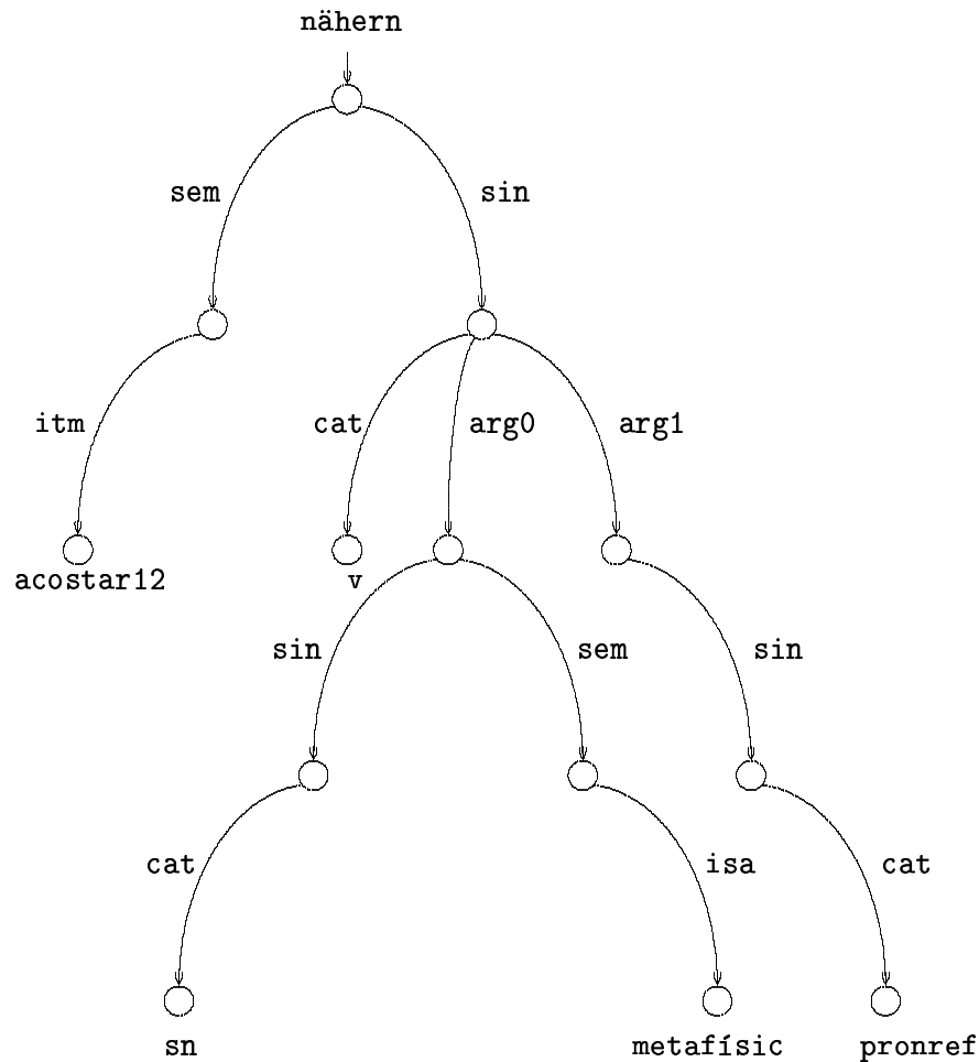
Figura 1.3: Graf corresponent a un dels usos del verb sich nähern .
