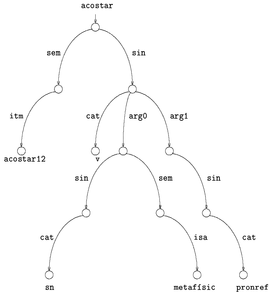
Figura 1.1: Graf corresponent a un dels usos del verb acostar .
