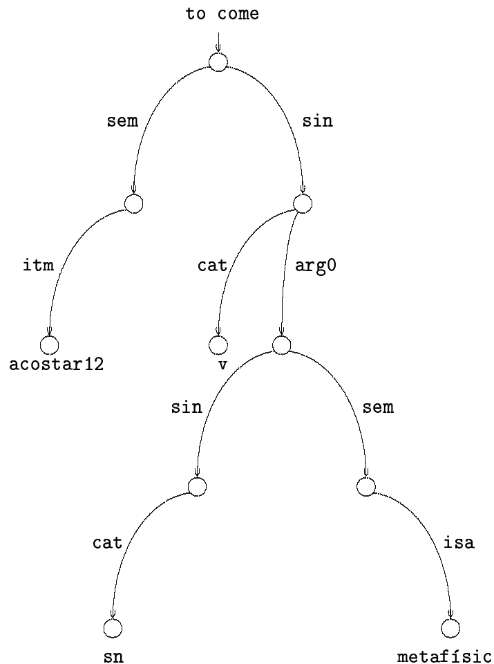
Figura 1.2: Graf corresponent a un dels usos del verb to come .
